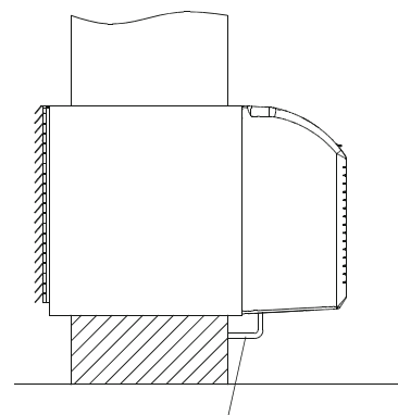
CHEMINEMENT DU CÂBLE DU THERMOSTAT (SOUS LE MANCHON, DERRIÈRE LE PANNEAU AVANT)
